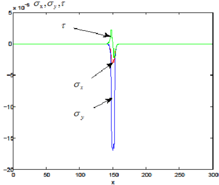
Рис. 1. – Нормальные и касательные напряжений в зависимости от координат и времени при x = 1dx - 255dx , y = 8dy , t = 251dt
