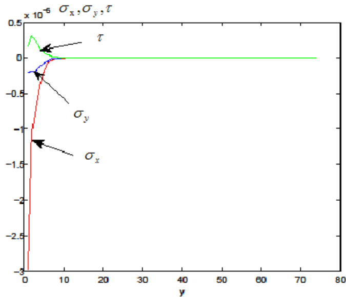
Рис. 3. – Нормальные и касательные напряжений в зависимости от координат и времени при x=119dx , y=1dy-64dy , t=251dt
