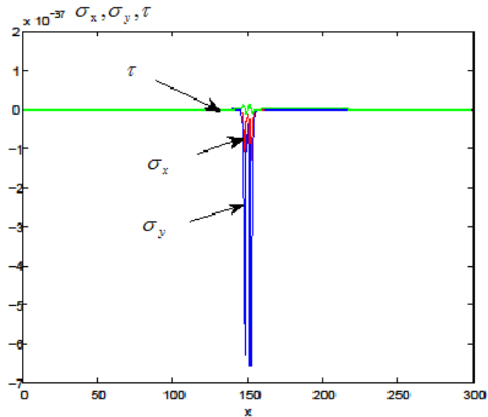
Рис. 2. – Нормальные и касательные напряжений в зависимости от координат и времени при x = 1dx - 255dx , y = 42dy , t = 251dt
