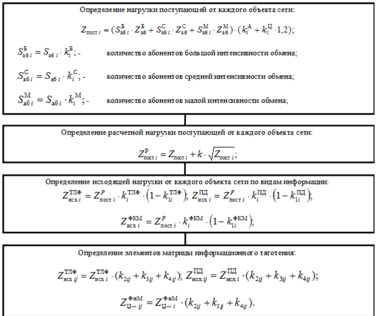
Рисунок 3. Блок-схема обобщенного алгоритма решения задачи расчета ожидаемых интенсивностей нагрузки и потоков вызовов в направлениях связи и формирования матрицы информационного тяготения.
